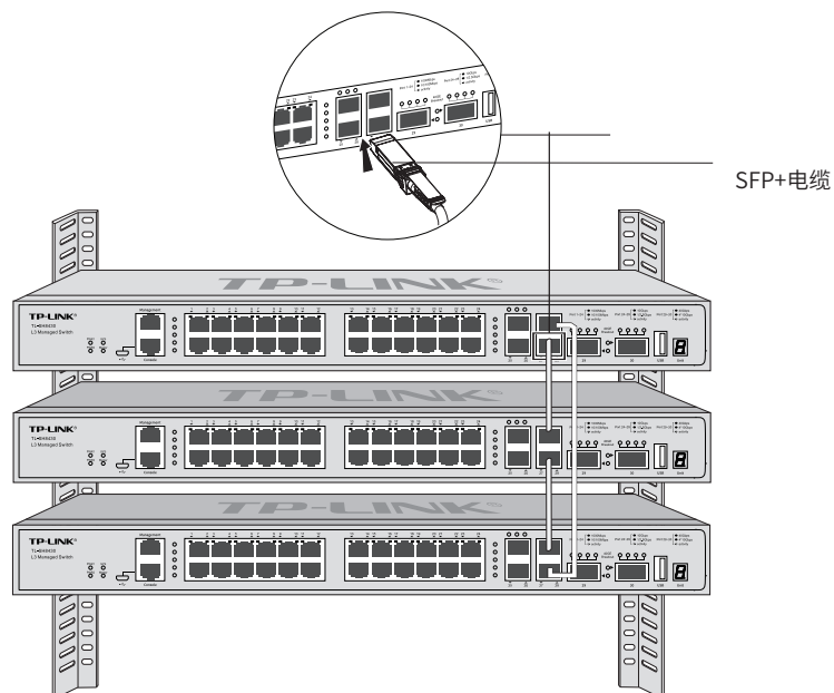
图2-4 使用SFP+端口建立堆叠示意图
