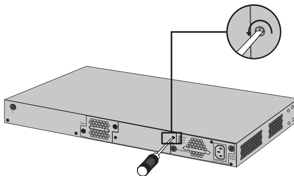
图3-6 移除保护面板示意图
