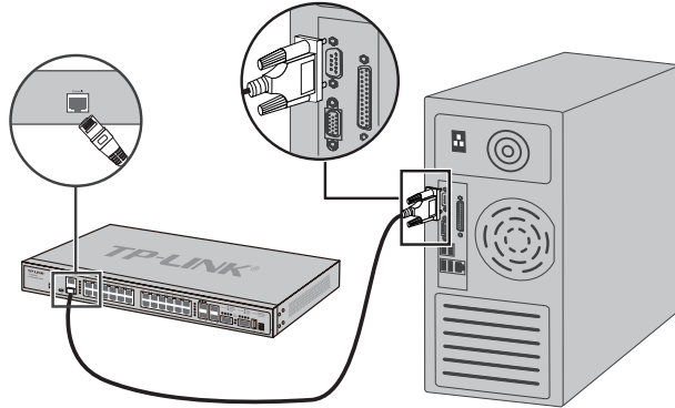
图3-3 RJ45 Console端口连接示意图
