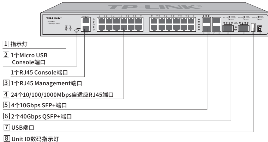
图1-1 TL-SH8430前面板示意图
